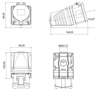
ГАБАРИТНЫЙ ЧЕРТЁЖ
