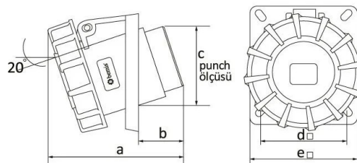
ГАБАРИТНЫЙ ЧЕРТЁЖ
