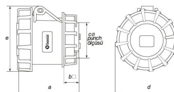
ГАБАРИТНЫЙ ЧЕРТЁЖ
