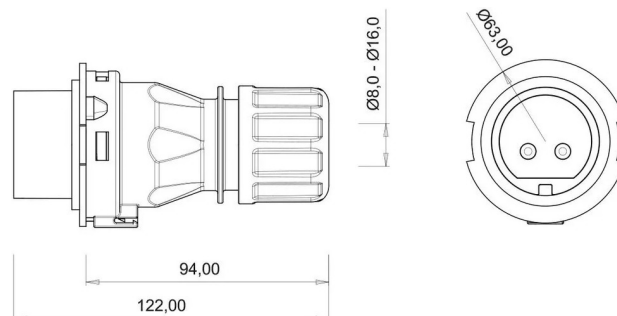
ГАБАРИТНЫЙ ЧЕРТЁЖ
