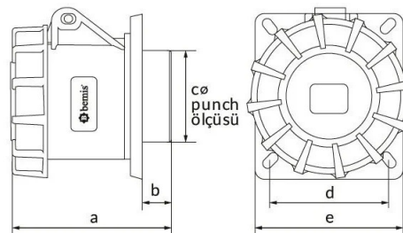
ГАБАРИТНЫЙ ЧЕРТЁЖ
