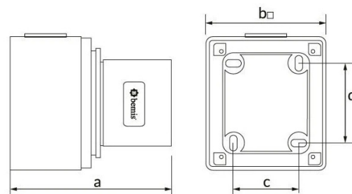
ГАБАРИТНЫЙ ЧЕРТЁЖ
