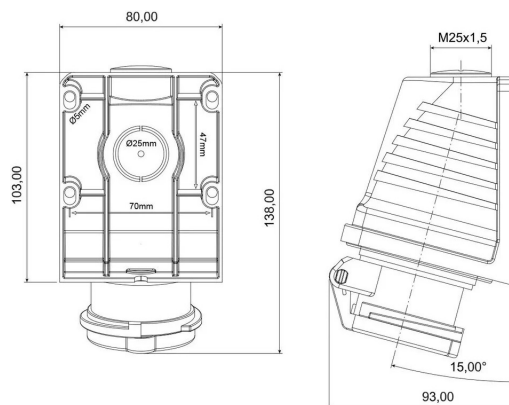
ГАБАРИТНЫЙ ЧЕРТЁЖ
