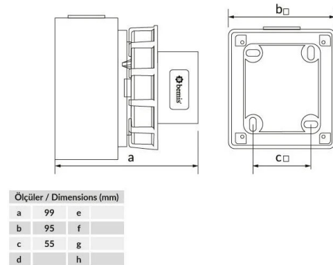
ГАБАРИТНЫЙ ЧЕРТЁЖ
