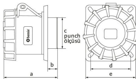
ГАБАРИТНЫЙ ЧЕРТЁЖ
