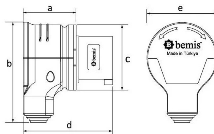
ГАБАРИТНЫЙ ЧЕРТЁЖ
