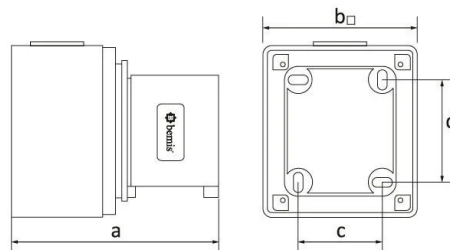
ГАБАРИТНЫЙ ЧЕРТЁЖ
