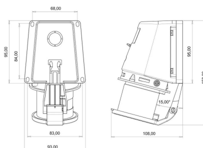
ГАБАРИТНЫЙ ЧЕРТЁЖ
