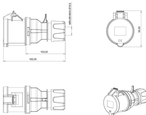
ГАБАРИТНЫЙ ЧЕРТЁЖ
