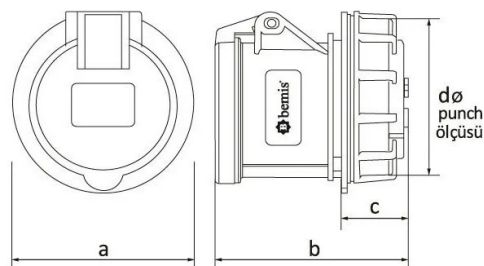
ГАБАРИТНЫЙ ЧЕРТЁЖ
