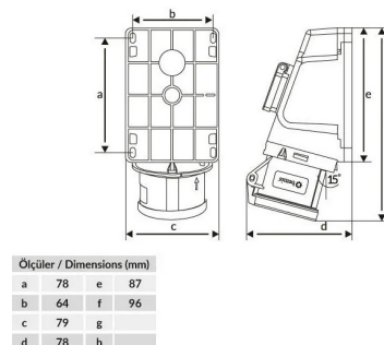
ГАБАРИТНЫЙ ЧЕРТЁЖ
