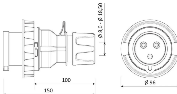
ГАБАРИТНЫЙ ЧЕРТЁЖ
