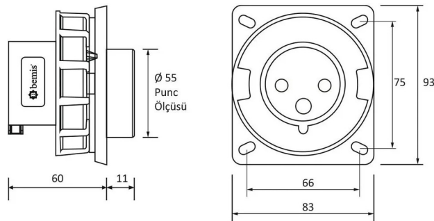
ГАБАРИТНЫЙ ЧЕРТЁЖ
