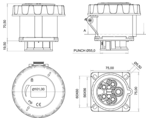
ГАБАРИТНЫЙ ЧЕРТЁЖ
