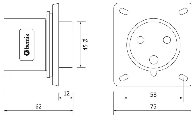
ГАБАРИТНЫЙ ЧЕРТЁЖ
