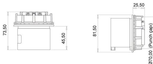
ГАБАРИТНЫЙ ЧЕРТЁЖ
