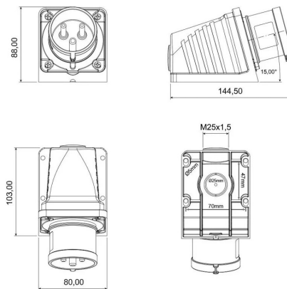
ГАБАРИТНЫЙ ЧЕРТЁЖ
