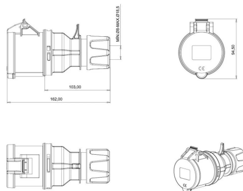
ГАБАРИТНЫЙ ЧЕРТЁЖ
