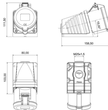
ГАБАРИТНЫЙ ЧЕРТЁЖ
