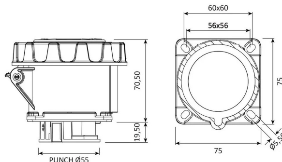
ГАБАРИТНЫЙ ЧЕРТЁЖ
