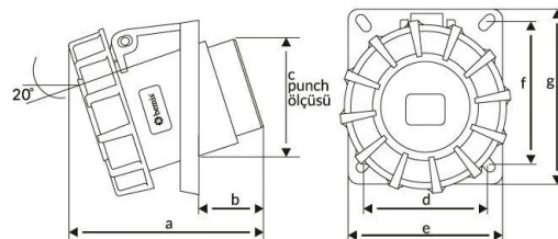
ГАБАРИТНЫЙ ЧЕРТЁЖ
