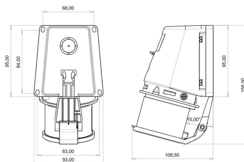
ГАБАРИТНЫЙ ЧЕРТЁЖ
