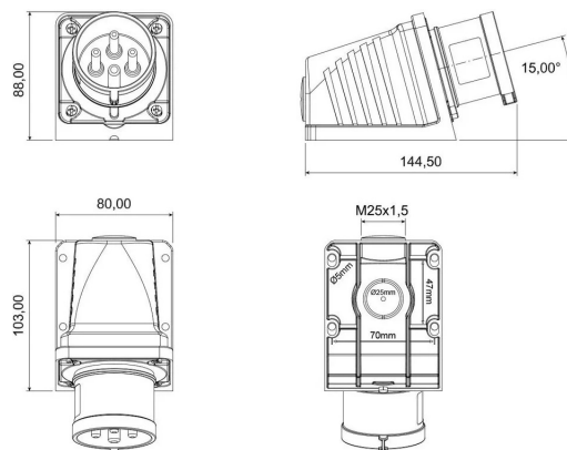
ГАБАРИТНЫЙ ЧЕРТЁЖ
