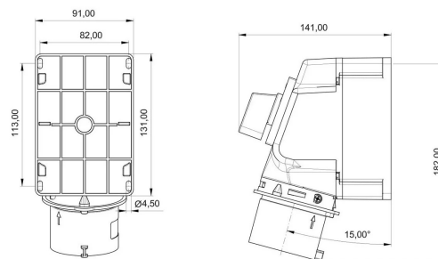
ГАБАРИТНЫЙ ЧЕРТЁЖ
