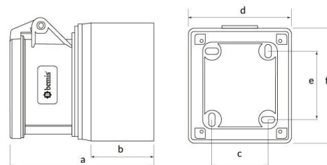
ГАБАРИТНЫЙ ЧЕРТЁЖ
