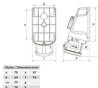
ГАБАРИТНЫЙ ЧЕРТЁЖ
