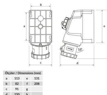
ГАБАРИТНЫЙ ЧЕРТЁЖ
