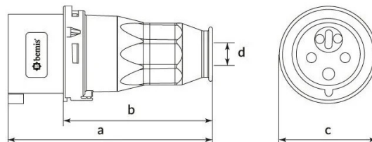
Ölçüler / Dimensions (mm)
