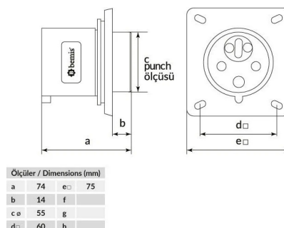
ГАБАРИТНЫЙ ЧЕРТЁЖ
