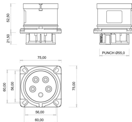
ГАБАРИТНЫЙ ЧЕРТЁЖ
