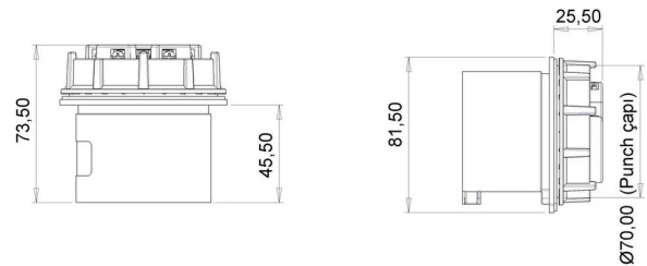
ГАБАРИТНЫЙ ЧЕРТЁЖ
