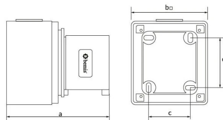
Ölçüler / Dimensions (mm)
