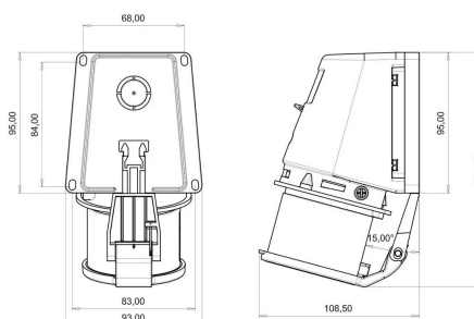
ГАБАРИТНЫЙ ЧЕРТЁЖ
