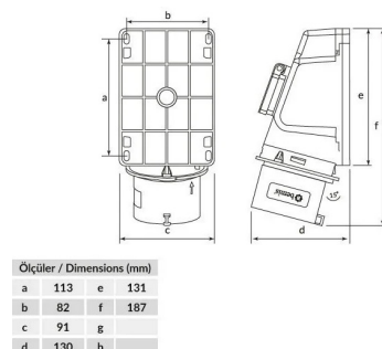
ГАБАРИТНЫЙ ЧЕРТЁЖ
