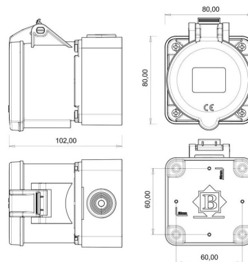
ГАБАРИТНЫЙ ЧЕРТЁЖ
