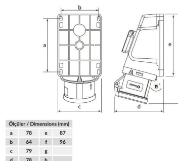
ГАБАРИТНЫЙ ЧЕРТЁЖ
