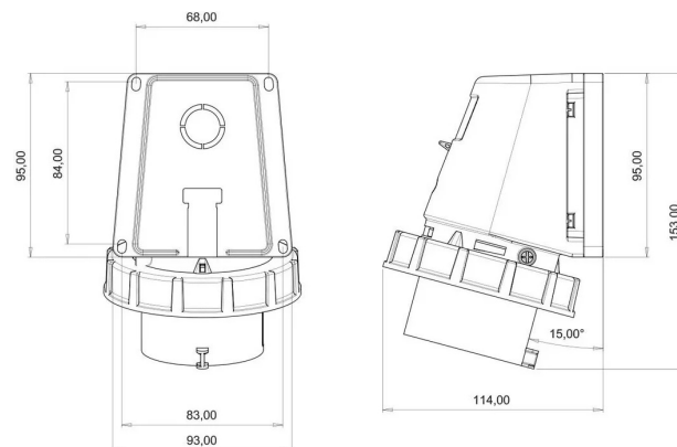
ГАБАРИТНЫЙ ЧЕРТЁЖ
