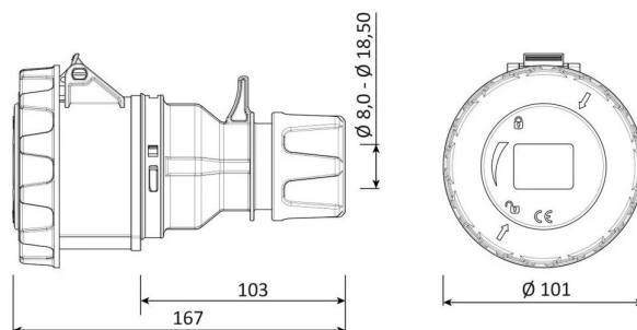
ГАБАРИТНЫЙ ЧЕРТЁЖ
