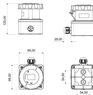
ГАБАРИТНЫЙ ЧЕРТЁЖ
