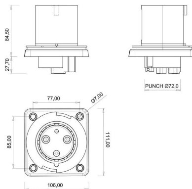
ГАБАРИТНЫЙ ЧЕРТЁЖ
