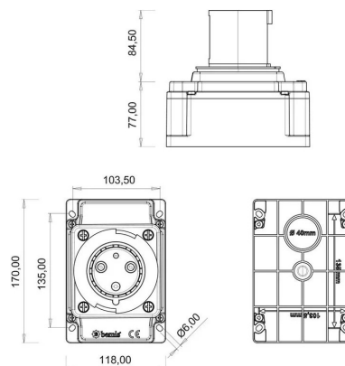
ГАБАРИТНЫЙ ЧЕРТЁЖ
