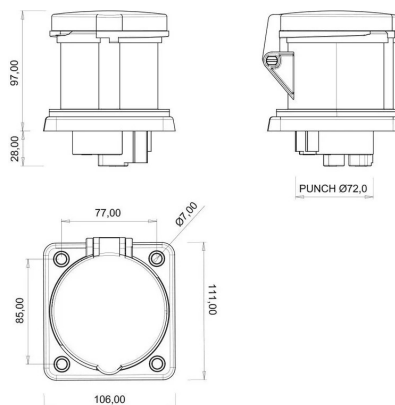
ГАБАРИТНЫЙ ЧЕРТЁЖ
