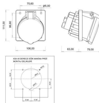
ГАБАРИТНЫЙ ЧЕРТЁЖ
