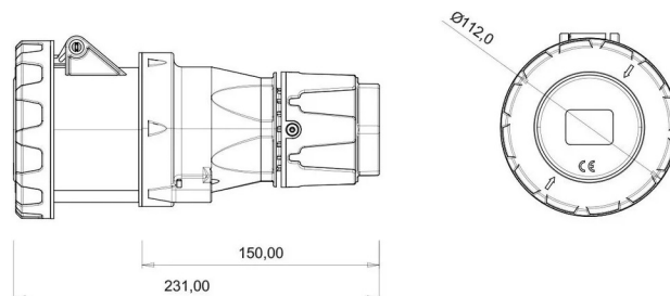
ГАБАРИТНЫЙ ЧЕРТЁЖ
