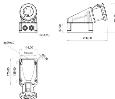
ГАБАРИТНЫЙ ЧЕРТЁЖ
