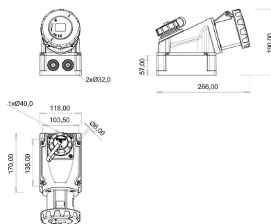
ГАБАРИТНЫЙ ЧЕРТЁЖ
